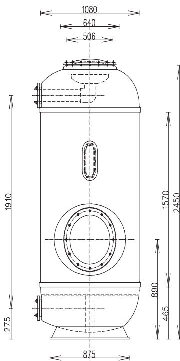
D 1080 H 2500 Flansch D 110 ART.-Nr. 0891931
