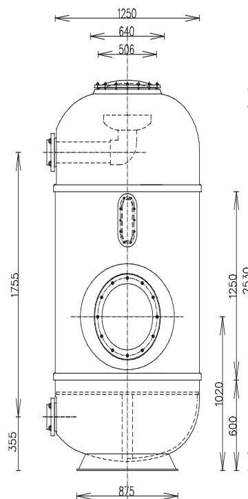
D 1250 H 2500 Flansch D 140 ART.-Nr. 0891932
