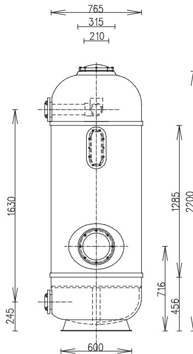
D 765 H 2200 Flansch D 90 ART.-Nr. 0891991
