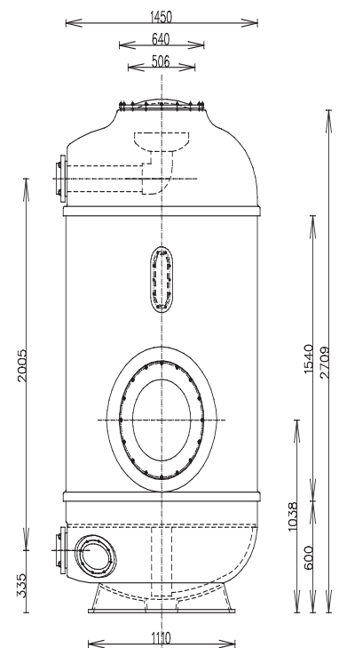
D 1450 H 2700 Flansch D 140 ART.-Nr. 0891933
