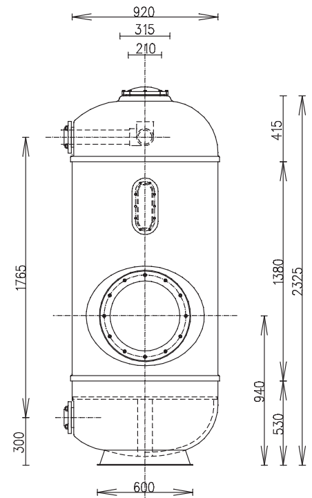
D 920 H 2350 Flansch D 90 ART.-Nr. 0891992
