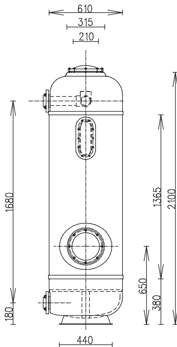
D 610 H 2100 Flansch D 75 ART.-Nr. 0891990
